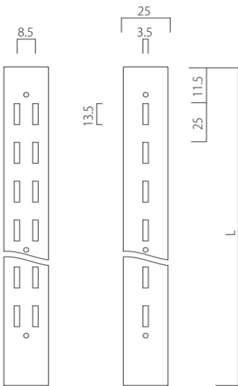
剖面圖
