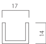
雙排 W14
