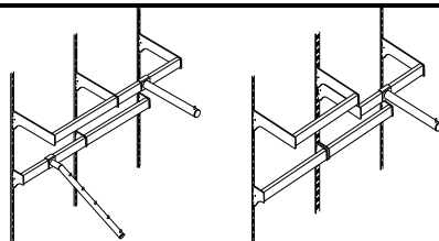
施工範例
